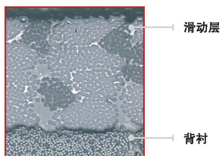
截面图
