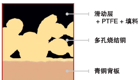
截面图
