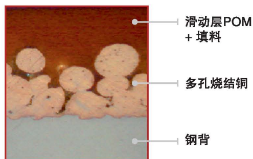
截面图
